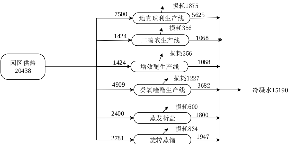
图 4.3-2 原料药厂区蒸汽平衡图 (t/a)
