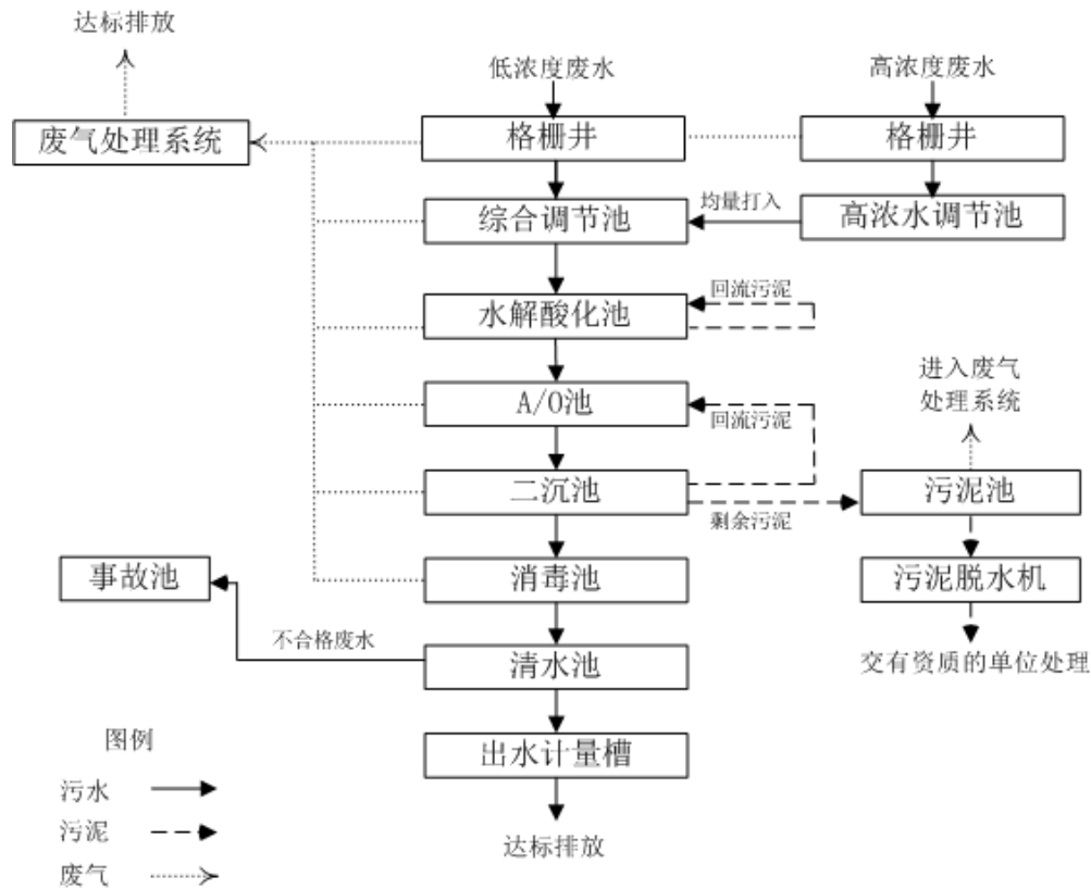
图 7.2.4-1 中华药港污水处理站工艺流程图
