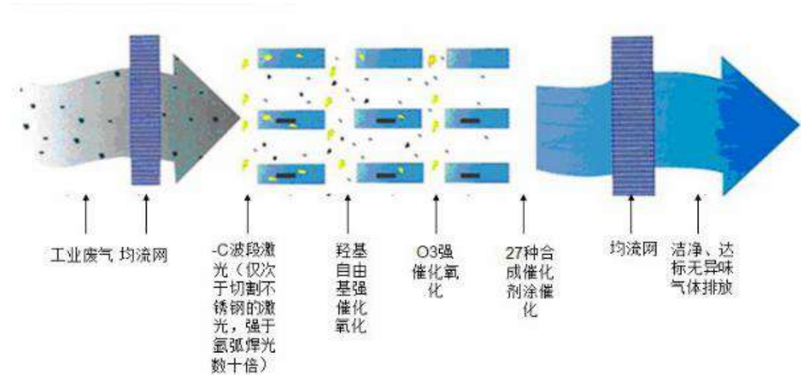
图 7.1.1-2 UV 光氧化处理原理示意图
