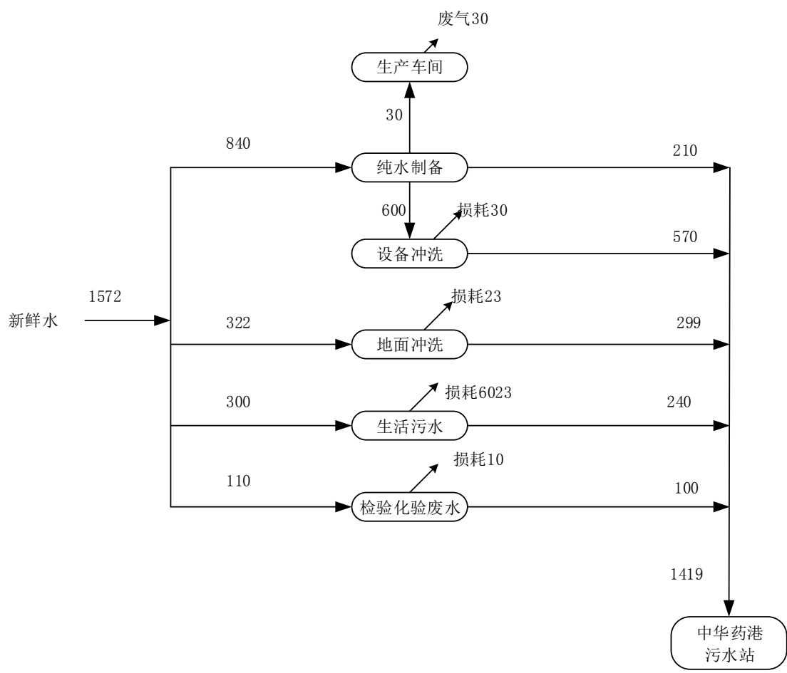
图 4.3-4 制剂厂区用水平衡图 (t/a)
