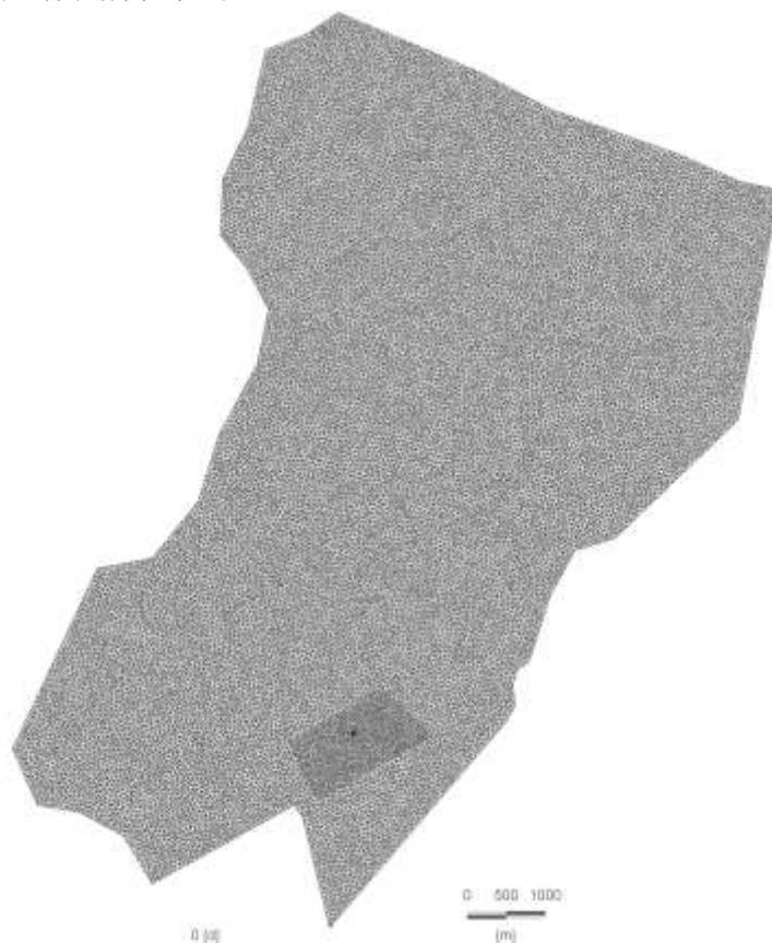
图 6.3-4 模型剖分图
