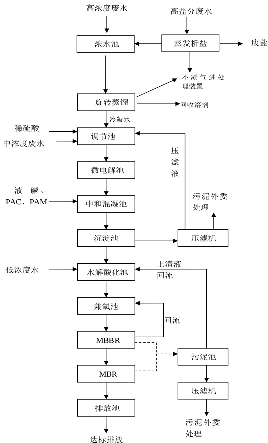
图 3.2-1 现有污水站废水处理工艺流程图
