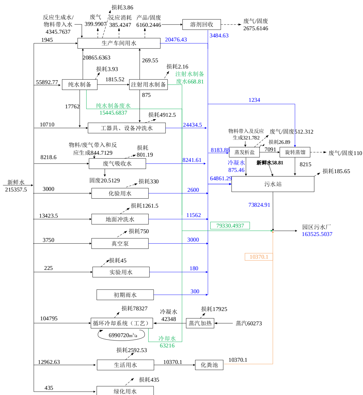
图 4.3-3 原料药厂区完成后全厂总用水平衡图 (t/a)
