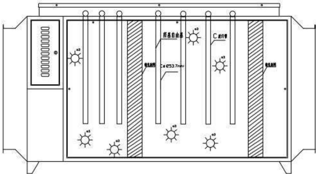
图 7.1.1-3 光氧化废气处理装置结构图
