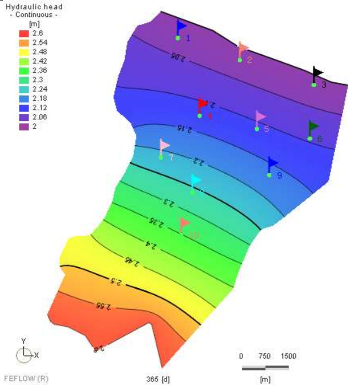
图 6.3-5 模拟计算流场图
