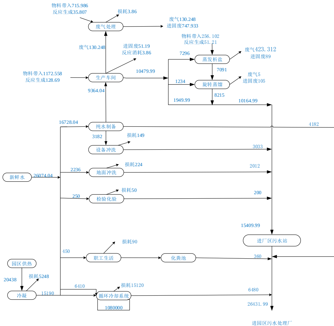
图 4.6-2 原料药厂区项目水平衡图 (t/a)
