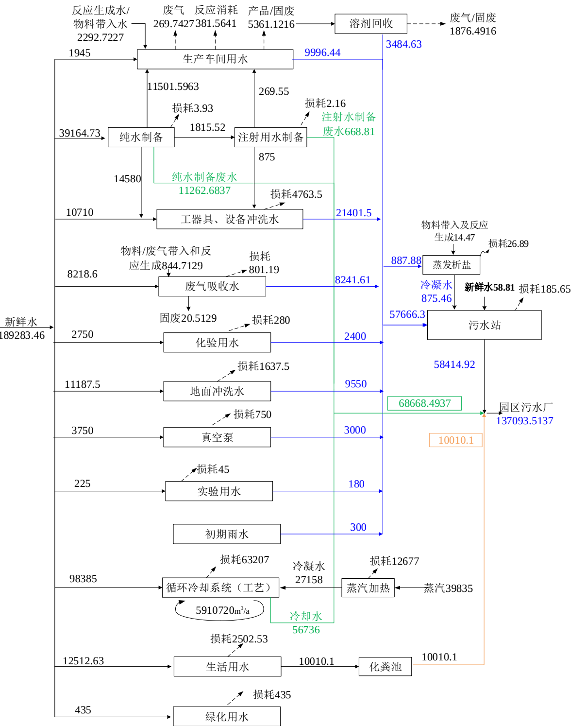
图 3.1-1 现有工程（已建+在建+拟建）给排水平衡图（单位：m³/a）
