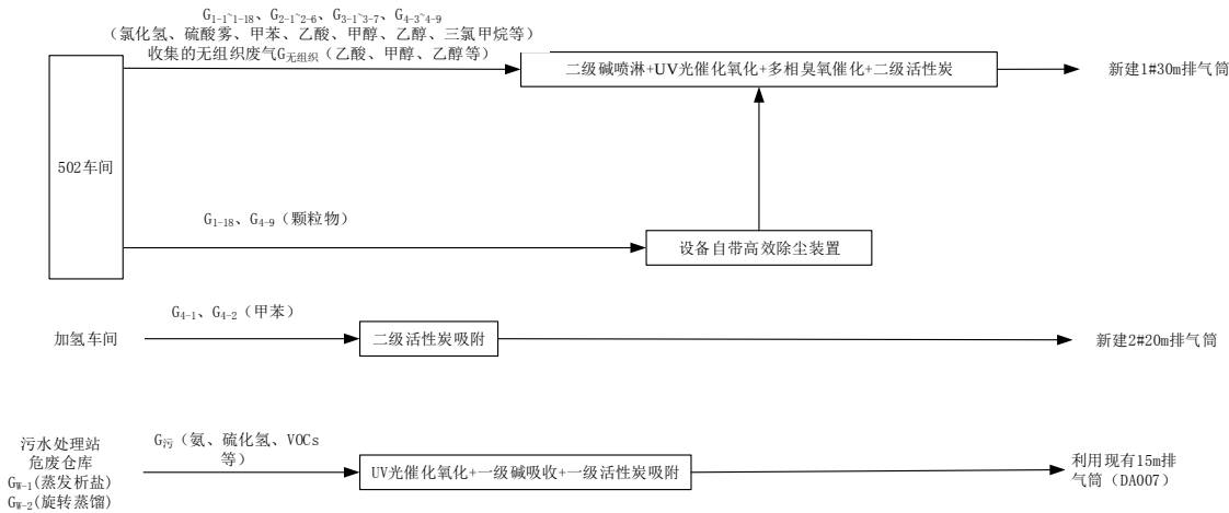
图 7.1.1-1 项目有组织废气污染物走向图
