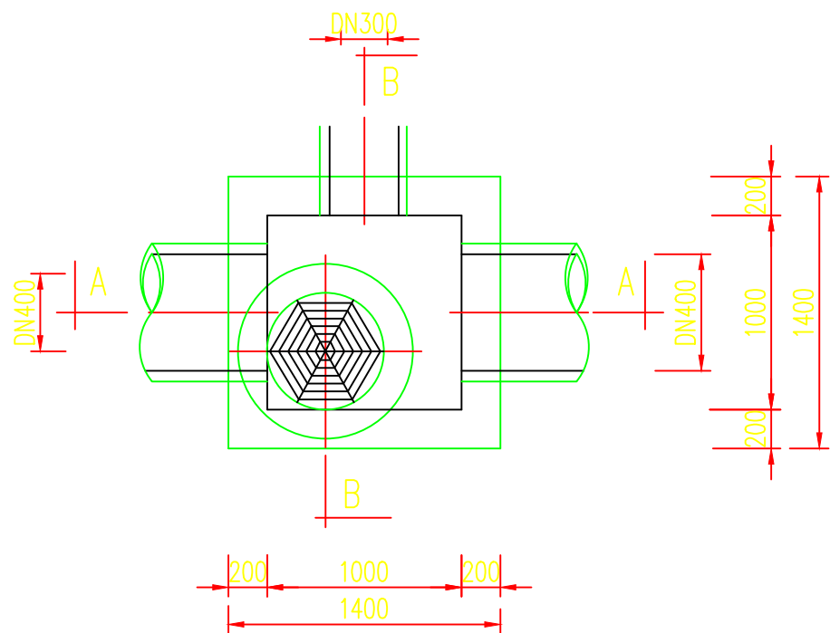
检查井平面图
