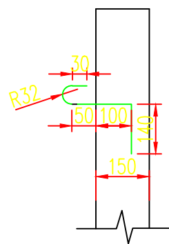
防坠网挂钩大样图
